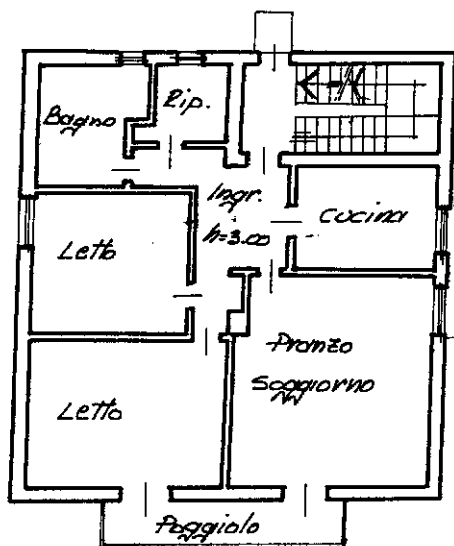
Piano Secondo
